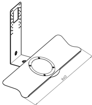
Tastaturadapter zur Montage am Monitor-Gelenkarm Best.-Nr.: 509205
