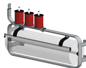
Aufsatz-Bandabroller für 3 Spulen Best.-Nr.: 124231
